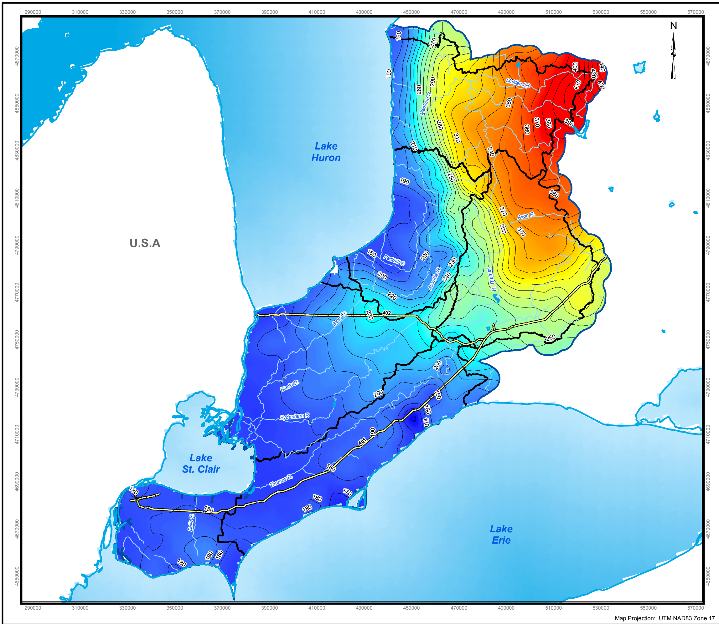
Figure 17: Bedrock Equipotentials
